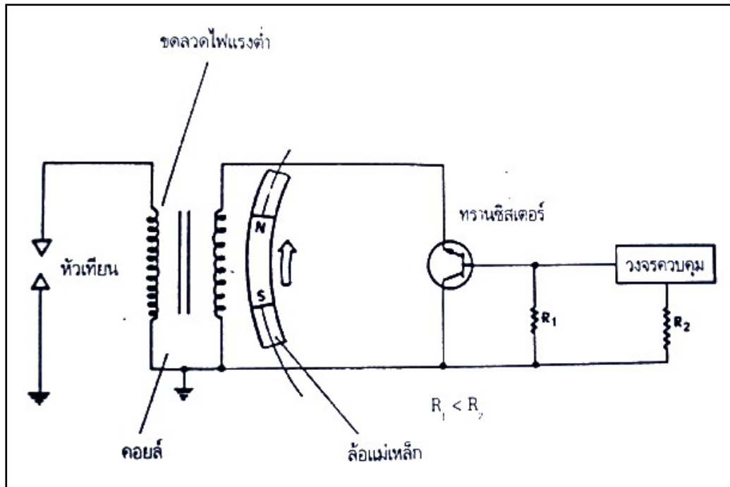
รูปที่ 4.3 ส่วนประกอบวงจรระบบจลน์ระบบเปิดแบบทรานซิสเตอร์
