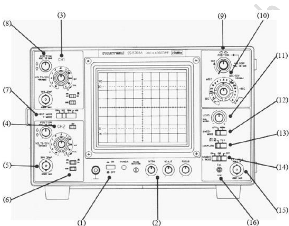
รูปที่ 2.6 แสดงออสซิลโลสโคป
