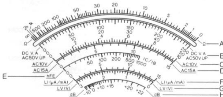
รูปที่ 2.2 แสดงสเกลการวัดของมัลติมิเตอร์
