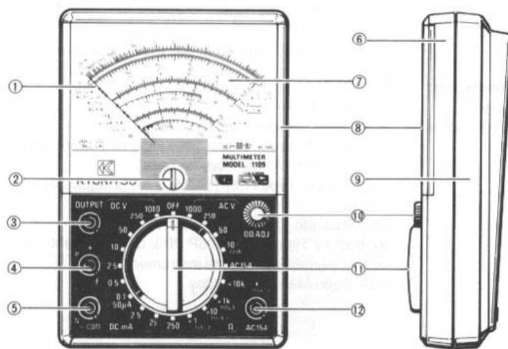
รูปที่ 2.1 แสดงลักษณะและส่วนประกอบของมัลติมิเตอร์
