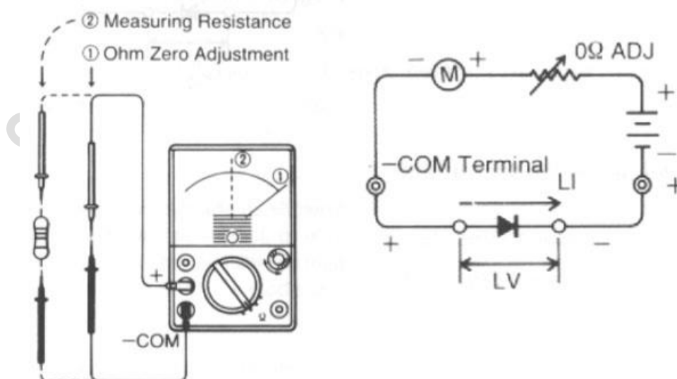
รูปที่ 2.4 แสดงโครงสร้างภายในของมิเตอร์ในขณะวัดค่าความต้านทาน
